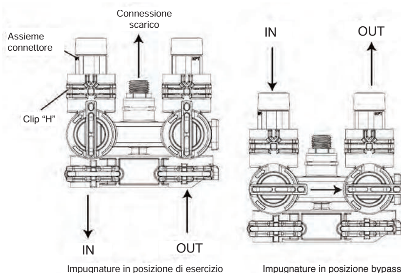
Figura 6 Funzionamento bypass
