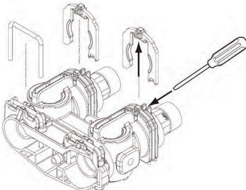
Figura 7 Assieme connettore
