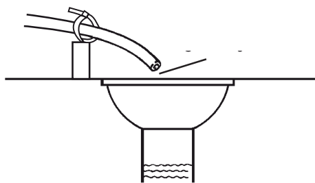
Figura 8 Conduttura di scarico con intercapedine d'aria
